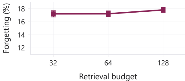
(d) Retrieval: forgetting
