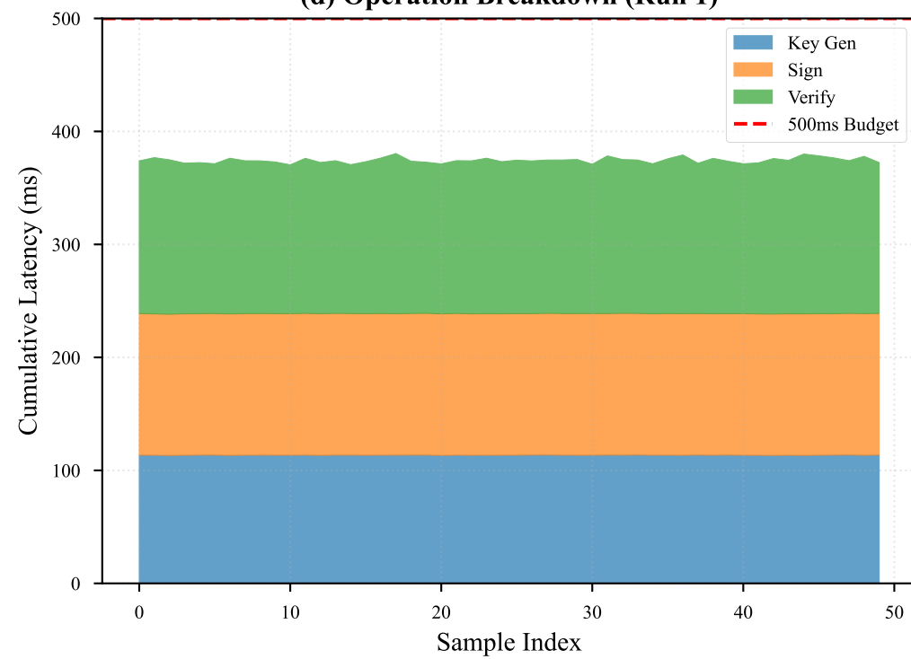
(d) Operation Breakdown (Run 1)
