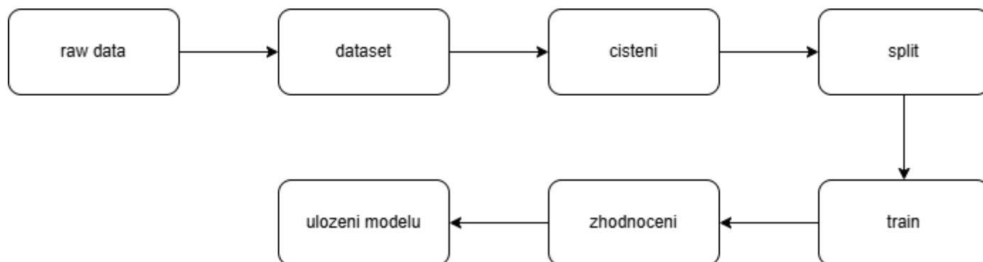
Diagram vývoje modelů
