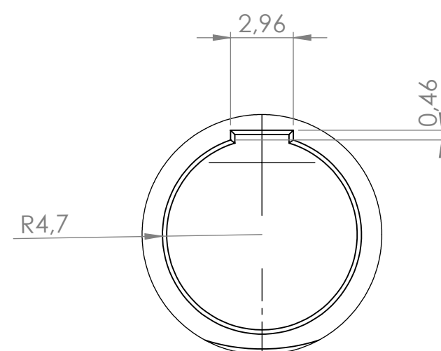
DETALLE B ESCALA 4 : 1
