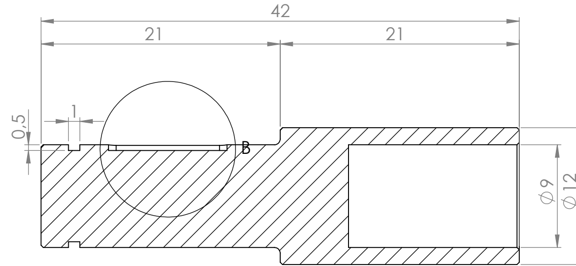
SECCIÓN A-A ESCALA 3 : 1
