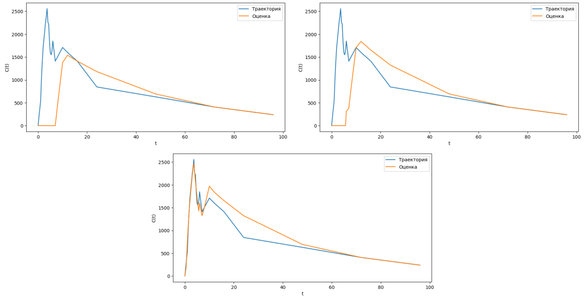
Рис. 4: Оценки построенные ансамблями из 1, 2 и 3 моделей с помощью пикового метода
