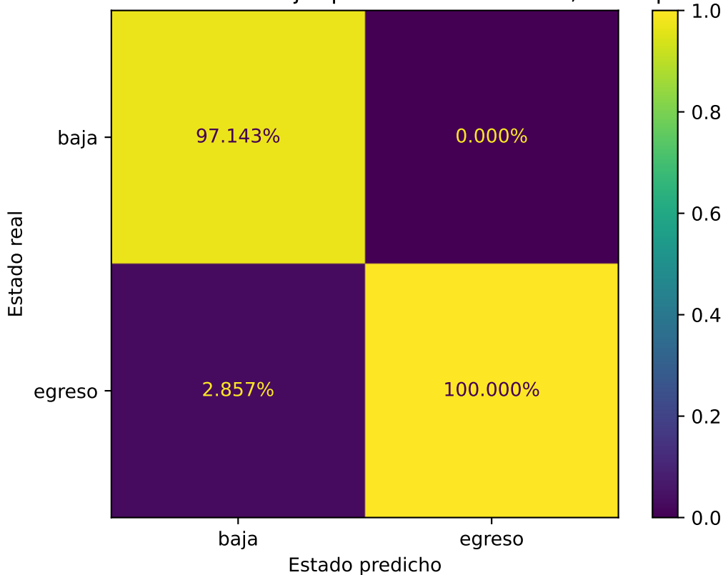
Matriz de confusion de la mejor prediccion de Estado, sobre predichos
