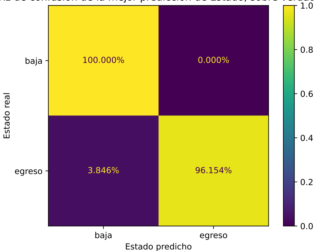
Matriz de confusion de la mejor prediccion de Estado, sobre verdaderos
