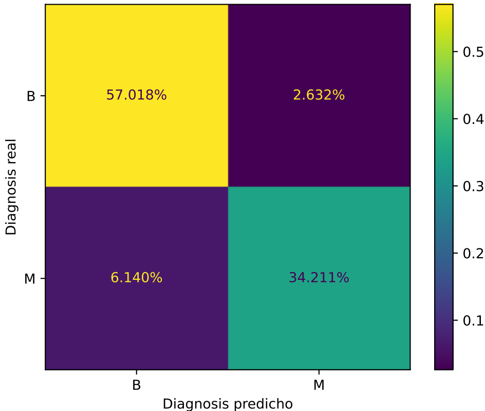
Matriz de confusion de Diagnosis, normalizado sobre all
