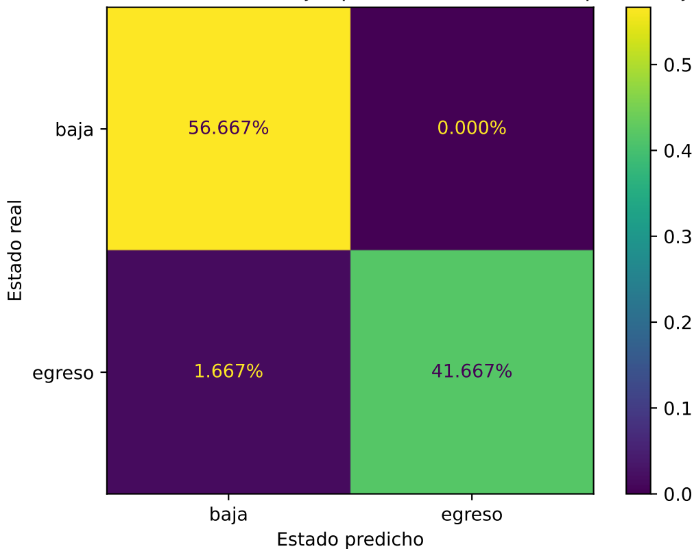
Matriz de confusion de la mejor prediccion de Estado, porcentajes
