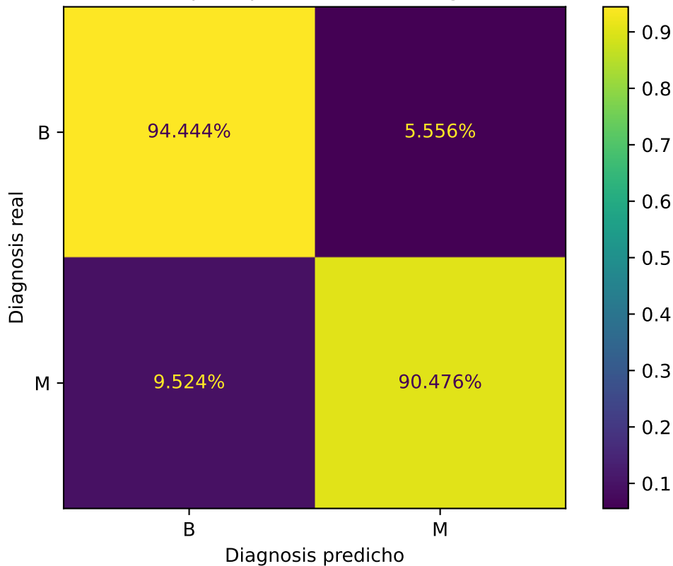
Matriz de confusion de la peor prediccion de Diagnosis, sobre verdaderos
