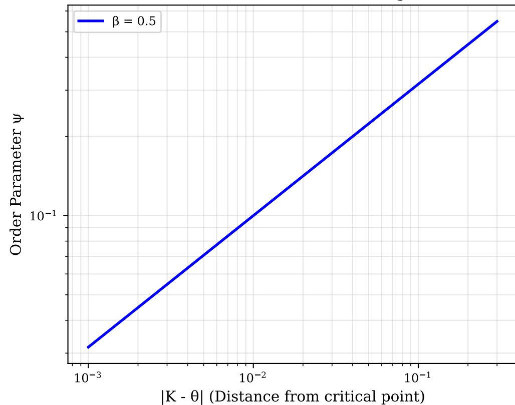
A) Order Parameter Scaling
