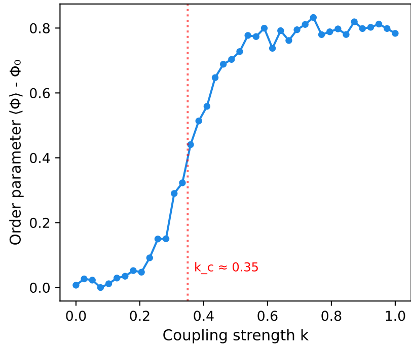
(a) Order Parameter
