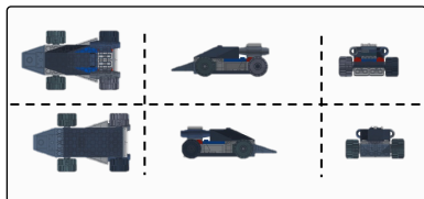
GPT-5.4
