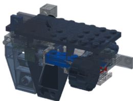
GPT-5.4
