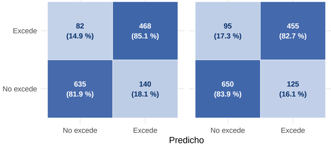
Logística (umbral 0.273)
