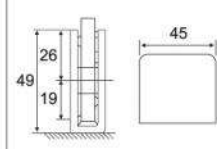
ECN-1153 مشبك تثبيت 0 درجة بفتحة واحدة Fix clip 0° single hole
