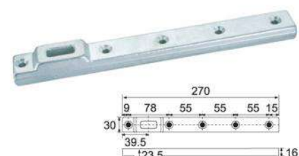
AC-06 مركز محوري الذراع Center Pivoted Arm
