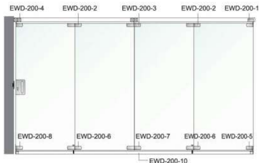
EWD-200-1 مشبك التثبيت العلوي Upper fixing clip
