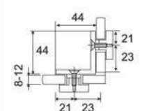
ECN-1096 مشبك تثبيت 90 درجة بفتحة مزدوجة Double 90°
