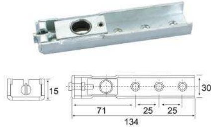
AC-01 مقعد محوري سفلي Pivot Bottom Seat
