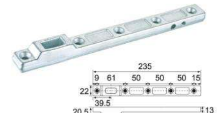
AC-07 مركز محوري الذراع Center Pivoted Arm
