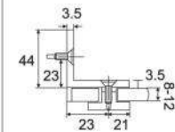
ECN-1095 مشبك تثبيت 90 درجة بفتحة واحدة Single 90°
