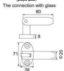
ESD-656 (دعامة زجاجية امامية ناتئة(توصيل كابل) Front cantilever glass bracket STD(cable connection)
