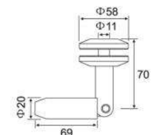
ESD-656 (دعامة زجاجية امامية ناتئة(توصيل كابل) Front cantilever glass bracket STD(cable connection)
