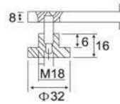
EHF-683 مخلب صغير بزاوية 90 درجة 90° Single spider
