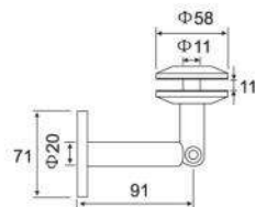
ESD-654 (وصلة جدار الي زجاج قياسية (وصلة كابل) Wall to glass connector STD(cable connection)
