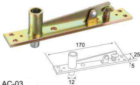
AC-03 مقعد محوري علوي Top Pivot Seat
