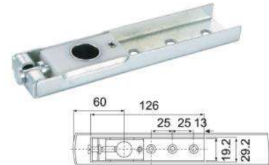
AC-04 مقعد محوري سفلي Pivot Bottom Seat
