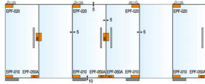
نمط مشبك الباب المربع Square patch fitting models
