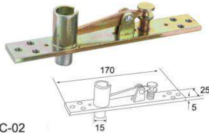
AC-02 مقعد محوري علوي Top Pivot Seat
