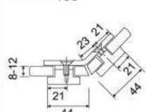
ECN-1098 مشبك تثبيت 135 درجة بفتحة مزدوجة Double 135°
