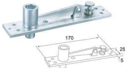
AC-04 مقعد محوري علوي Top Pivot Seat
