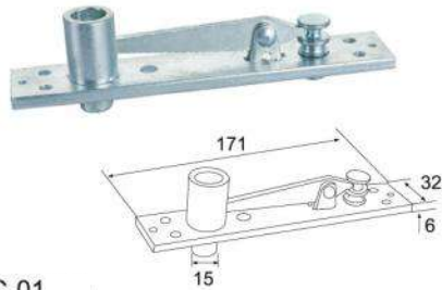
AC-01 مقعد محوري علوي Top Pivot Seat
