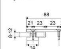
ECN-1099 مشبك تثبيت 180 درجة بفتحة واحدة Single 180°
