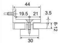
ECN-1094 مشبك تثبيت 0 درجة بفتحة مزدوجة Fix clip 0° double hole
