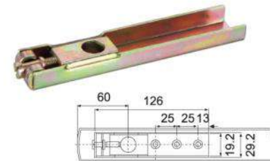
AC-03 مقعد محوري سفلي Pivot Bottom Seat
