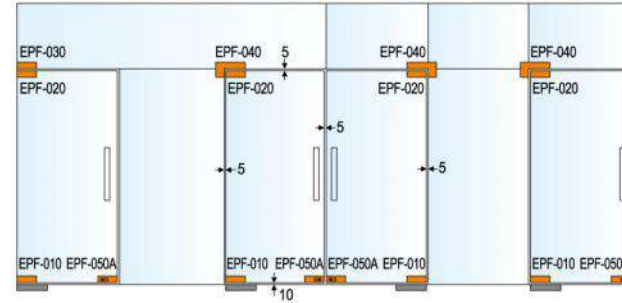
نمط مشبك الباب غير المنتظم Irregular patch fitting models
