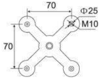
EHF-678 عنكبوت زجاجي بأربعة مخالب 4-Claw glass spider
