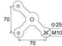
EHF-689 عنكبوت زجاجي بثلاثة مخالب 3-Claw glass spider
