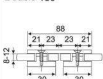
ECN-1100 مشبك تثبيت 180 درجة بفتحة مزدوجة Double 180°
