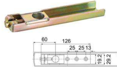
AC-02 مقعد محوري سفلي Pivot Bottom Seat
