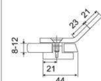
ECN-1097 مشبك تثبيت 135 درجة بفتحة واحدة Single 135°
