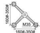
EJ-146 عنكبوت زجاجي على شكل حرف K K-Claw glass spider
