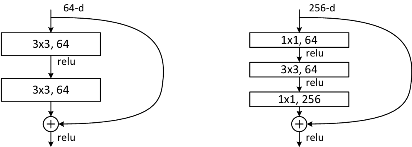
图 5. 用于 ImageNet 的更深残差函数 FF。左：如图 3 所示，ResNet-34 中的构建模块（位于 56 \times 56 特征图上）。右：用于 ResNet-50/101/152 的“瓶颈”（bottleneck）构建模块。
