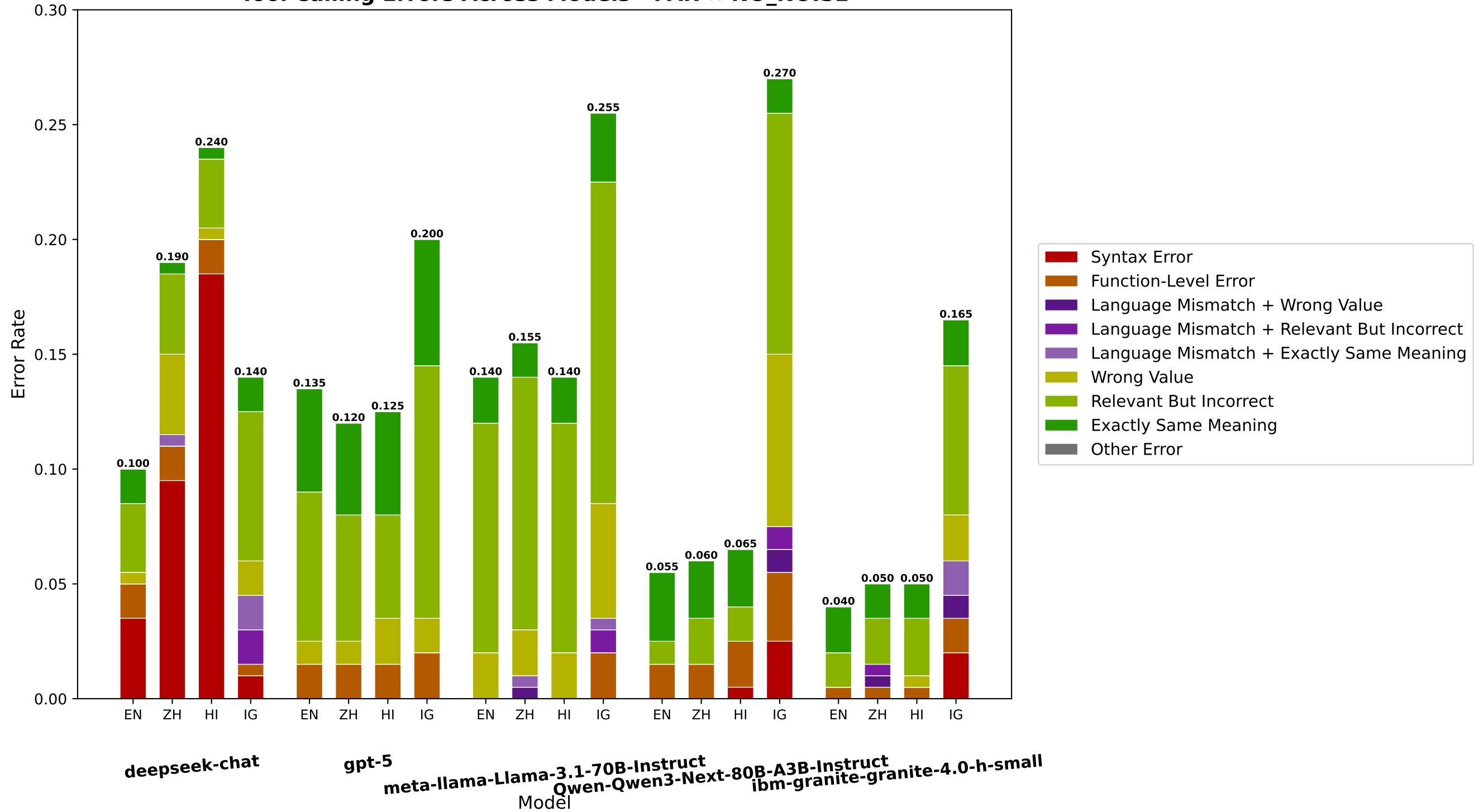
Tool Calling Errors Across Models - PAR × NO_NOISE
