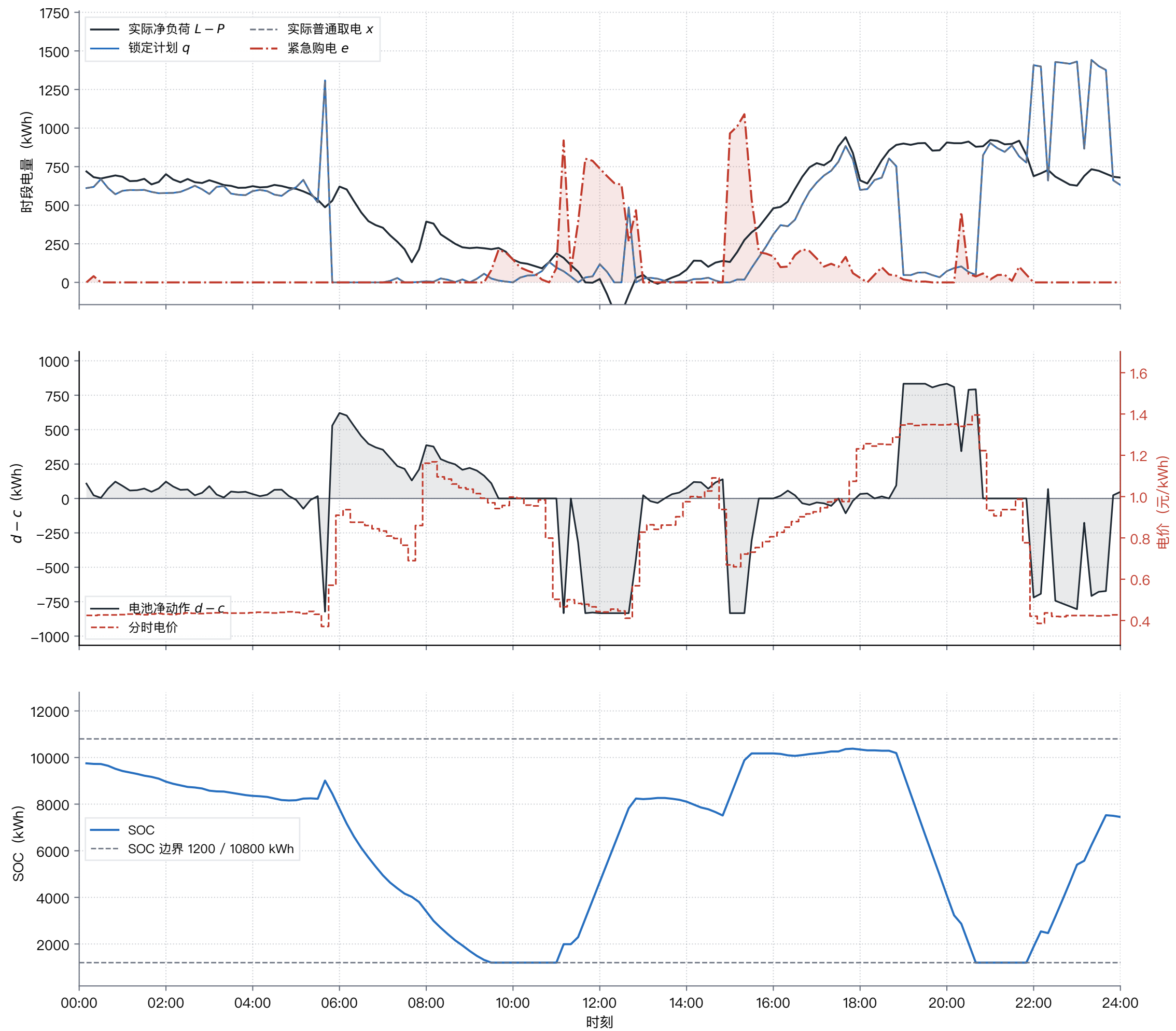
Q2 日前一日内联动轨迹：2025-06-01（紧急费用最高日）
