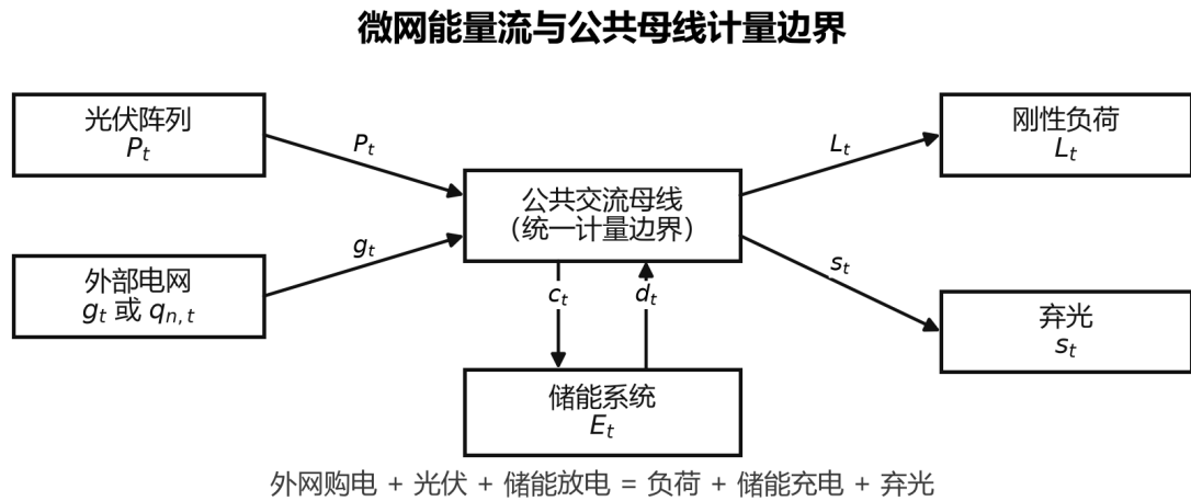
图2 微网能量流与公共母线计量边界
