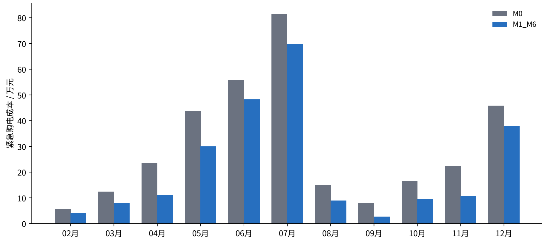
问题三 2025 年 2--12 月紧急购电成本月度对比
