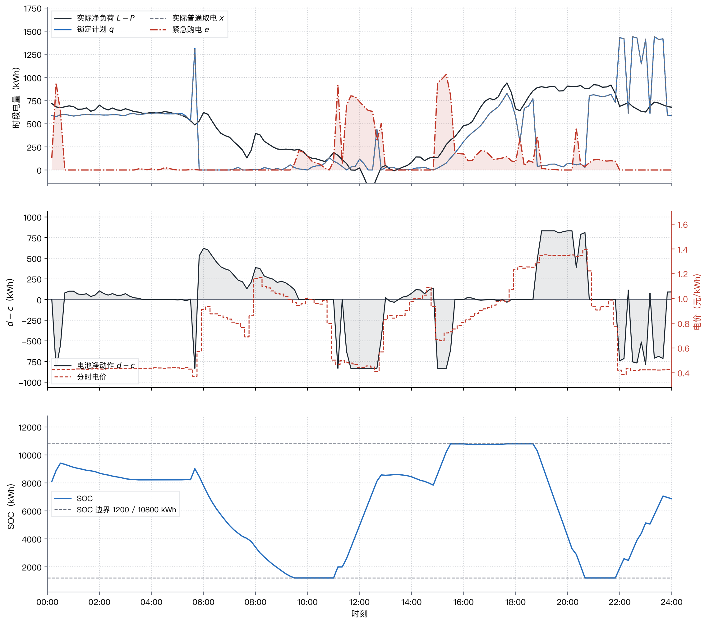
Q2 政策一致轨迹：2025-06-01 (2—12 月紧急费用最高日)
