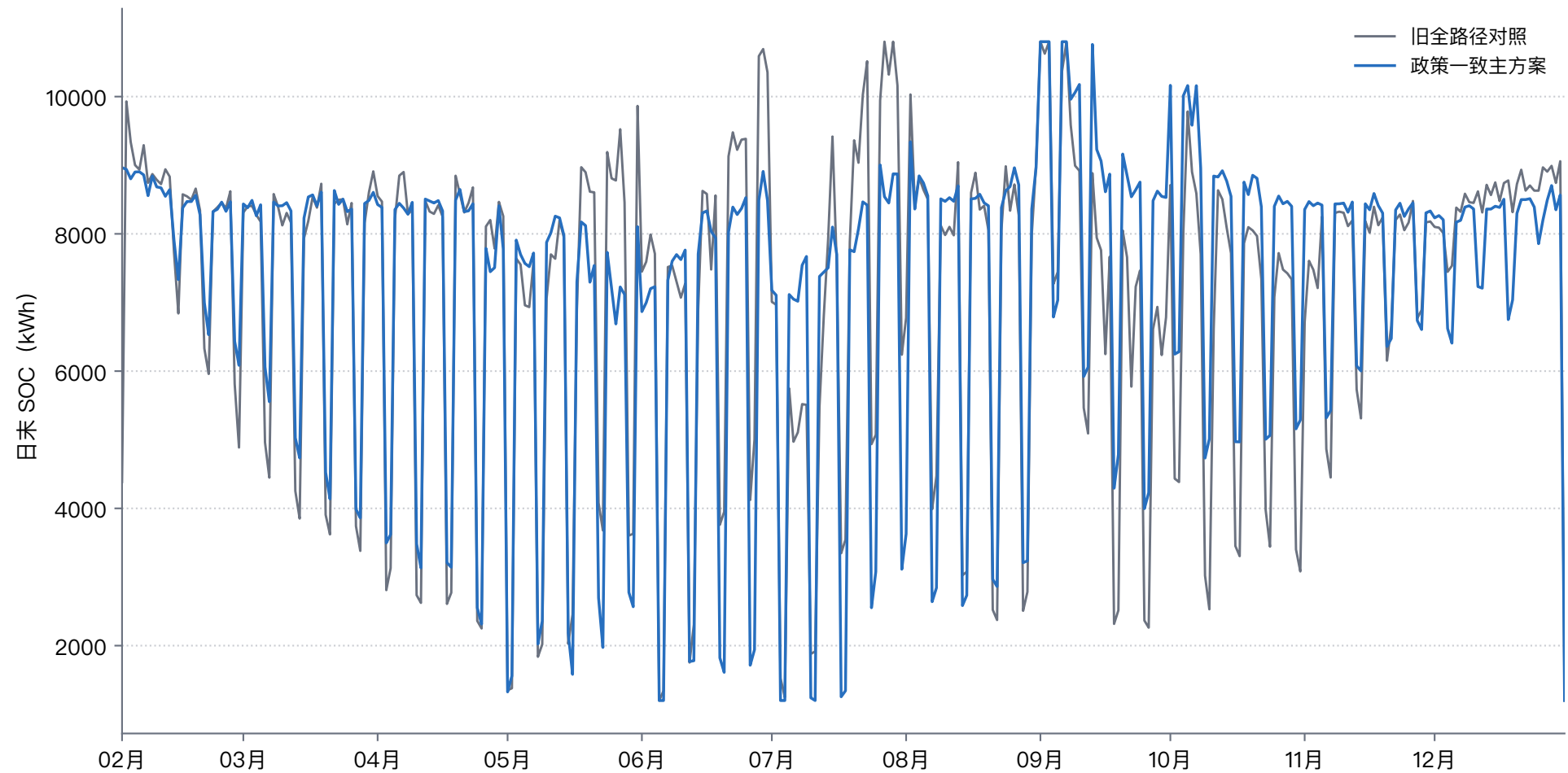
2—12 月储能日末 SOC 对照
