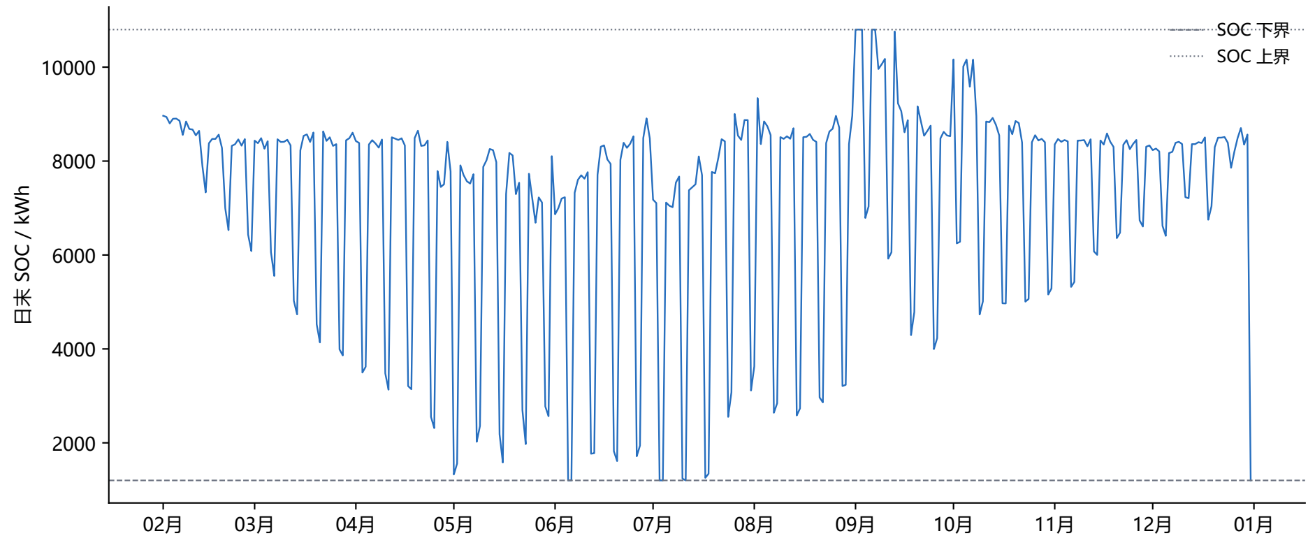
问题二 2025 年 2--12 月日末储电量轨迹
