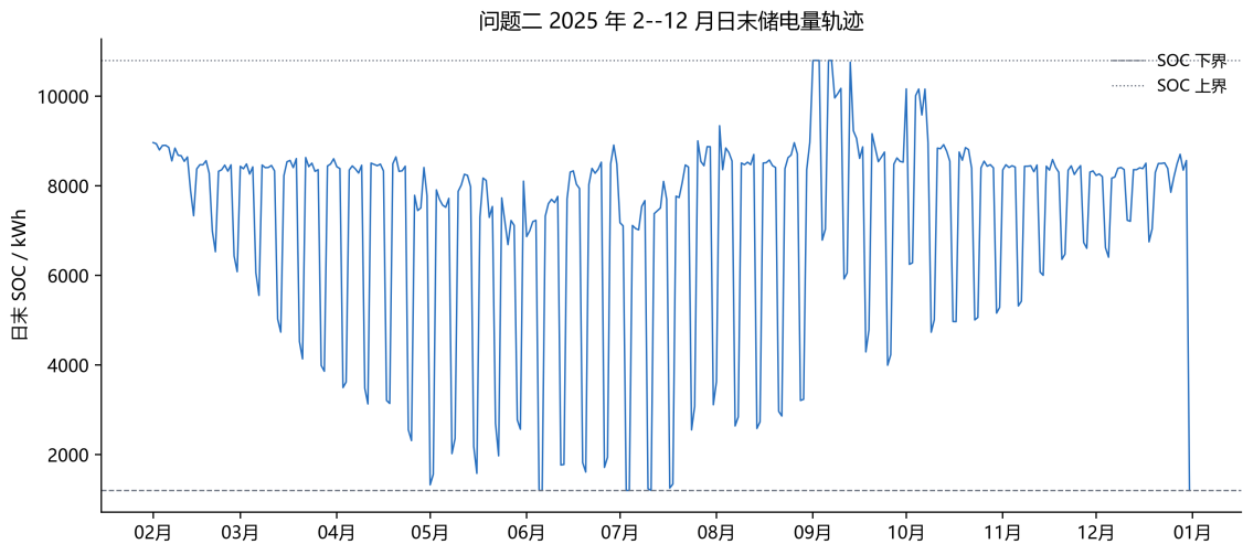
图 4 2025 年 2-12 月日末储电量轨迹; 虚线为 SOC 边界。
