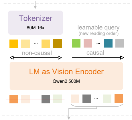
DeepEncoder V2
