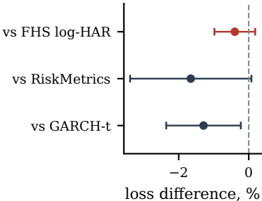
VaR/ES (FZ0)
