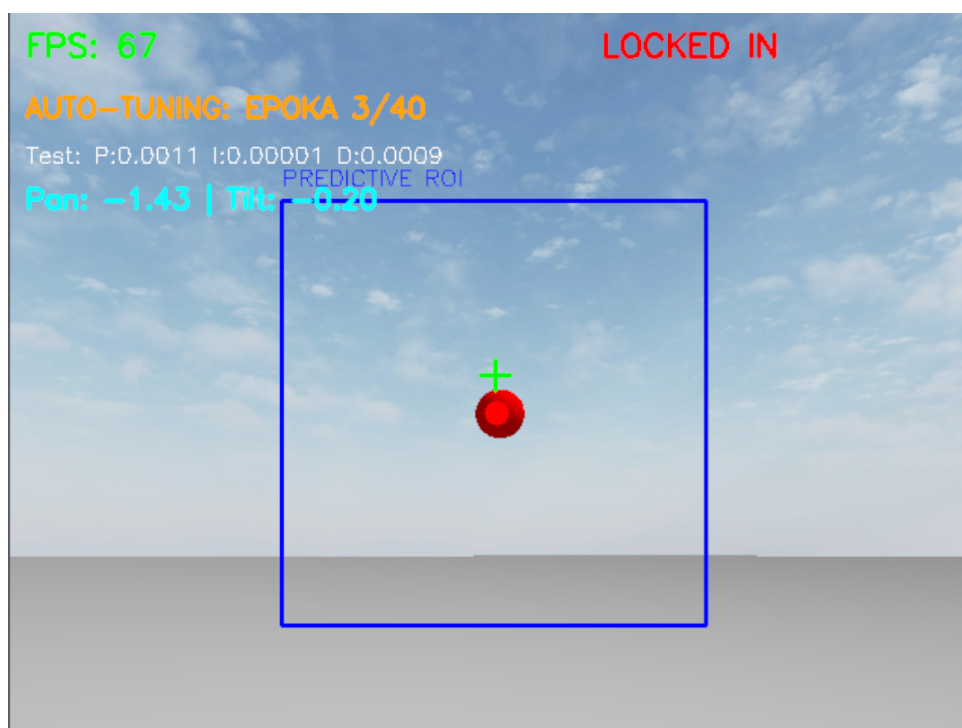
Rysunek 4.2: Interfejs nakładki diagnostycznej (OSD) w trybie auto-tuningu w środowisku symulacyjnym. Zrzut ekranu prezentuje 3 epokę uczenia, wyliczone na żywo kąty PAN/TILT oraz aktualne wartości nastaw regulatora PID weryfikowane na wykrytym i ograniczonym ramką obiekcie referencyjnym (Predictive ROI).
