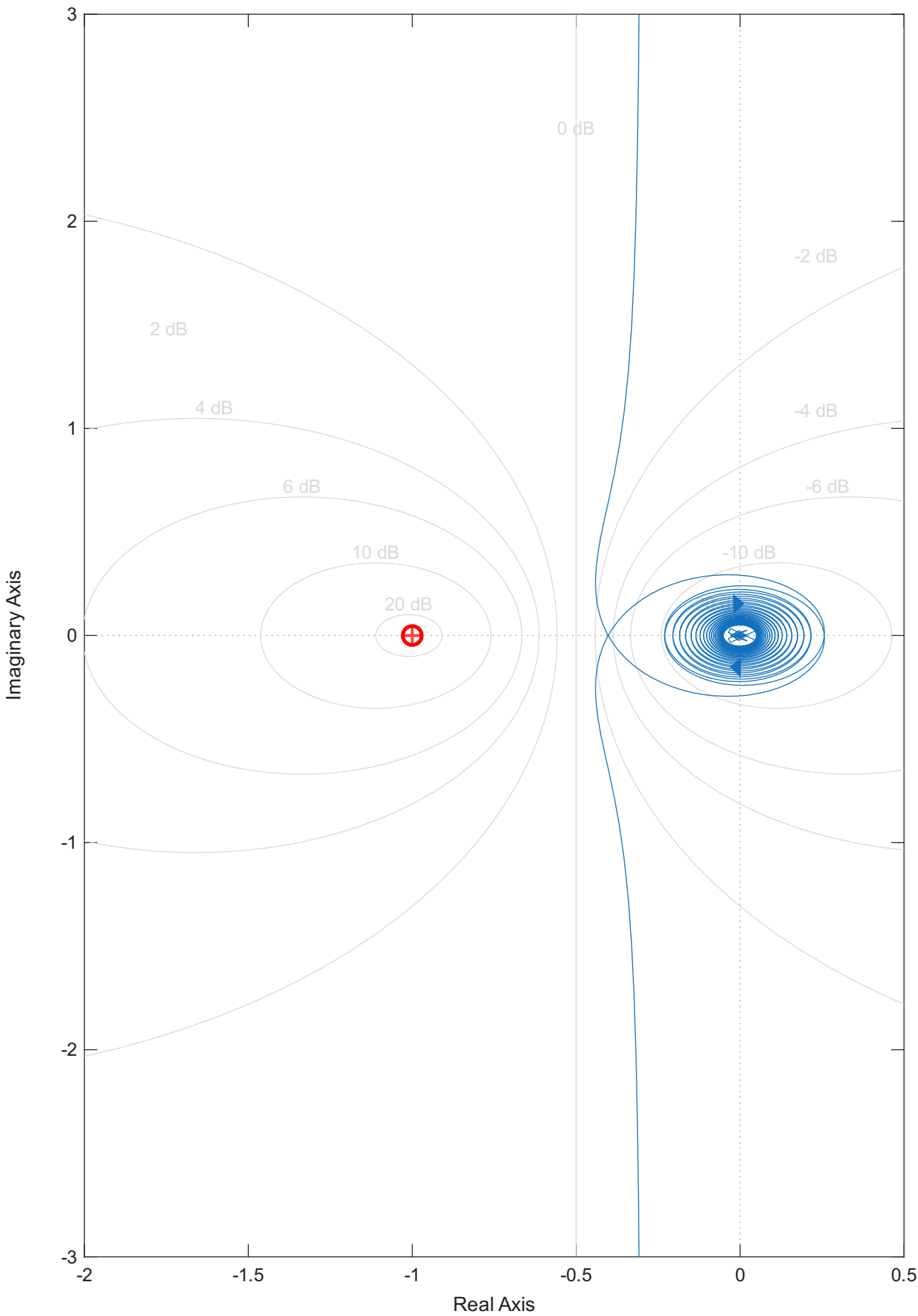
Nyquist-Diagramm des optimierten Regelkreises
