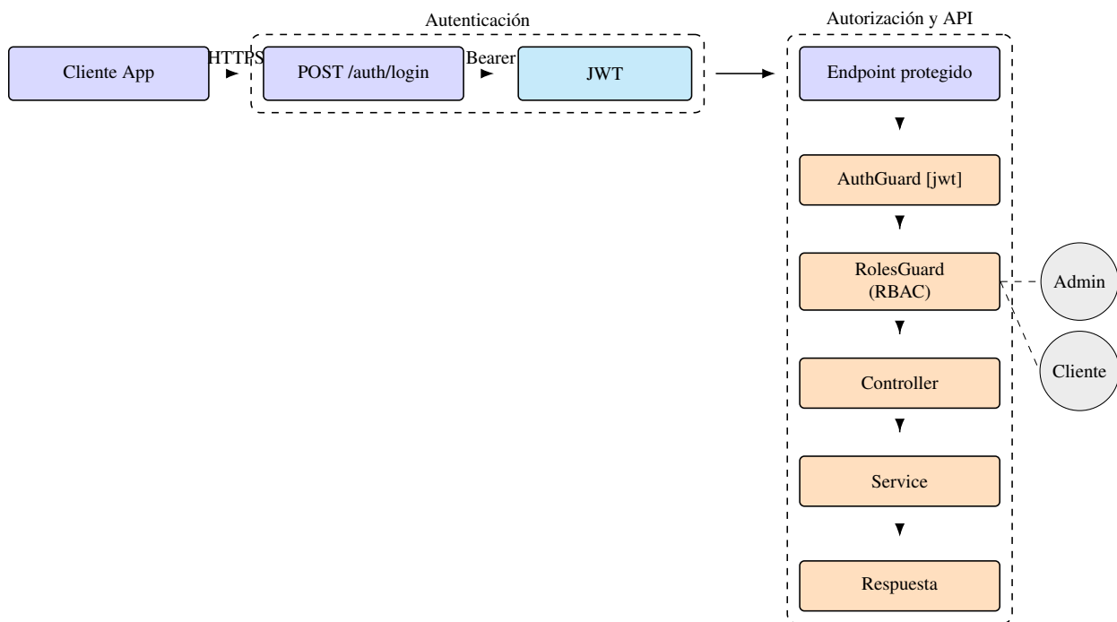
Figura 20. Flujo de autenticación y autorización (JWT + RBAC)
