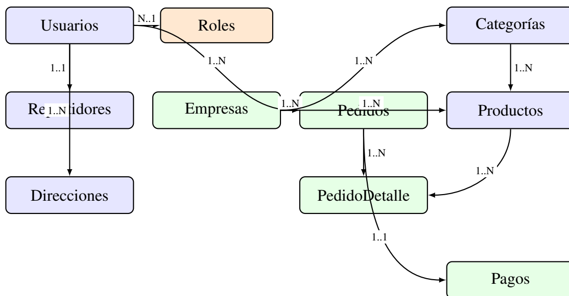
Figura 15. Diagrama entidad–relación de la base de datos de la plataforma SaaS
