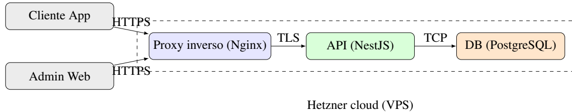
Figura 14. Arquitectura de despliegue (VPS, Vercel, APK)
