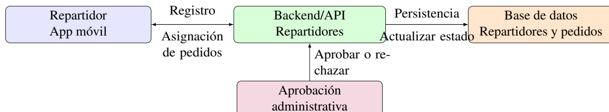
Figura 14. Diagrama del módulo de repartidores
