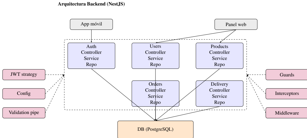
Figura 1. Arquitectura modular del backend (NestJS) planificada
