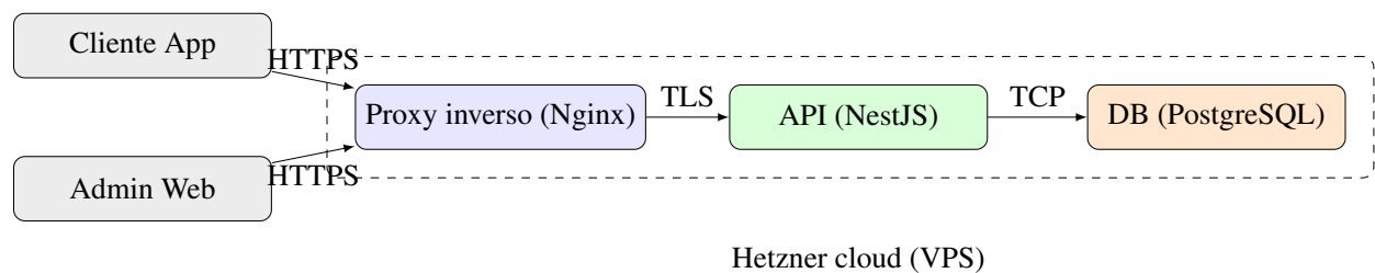
Figura 8. Arquitectura del despliegue de la plataforma
