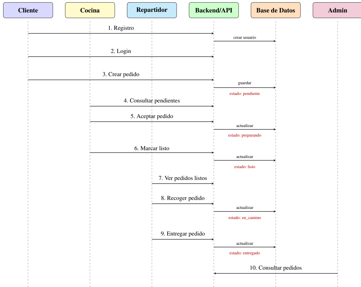
Figura 11. Diagrama de secuencia: flujo completo del proceso de pedido
