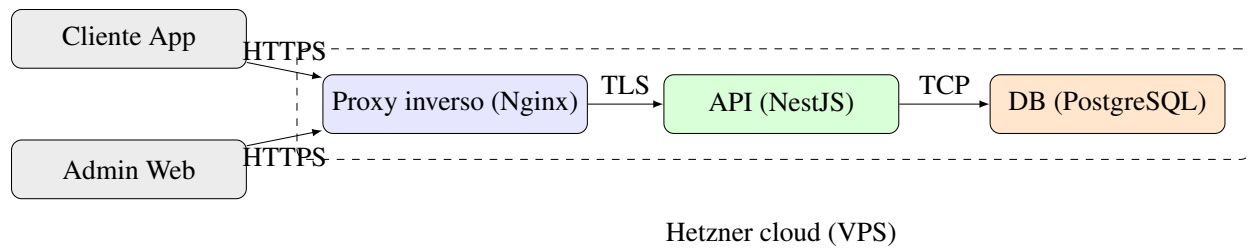
Figura 14. Arquitectura de despliegue (VPS, Vercel, APK)
