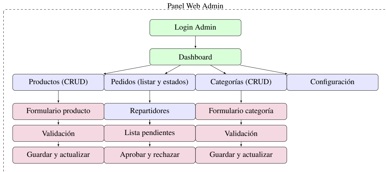
Figura 10. Flujo del panel web administrativo
