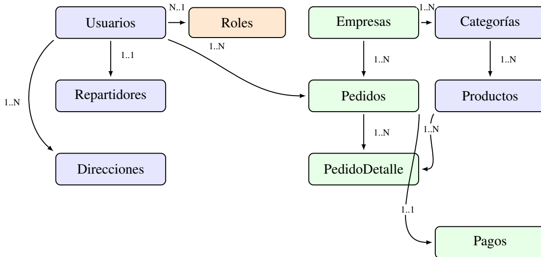
Figura 15. Diagrama entidad–relación de la base de datos de la plataforma SaaS
