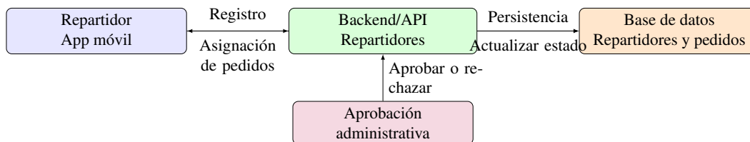
Figura 13. Diagrama de bloques del módulo de repartidores (versión ampliada en el Apéndice G)
