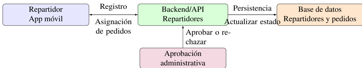
Figura 25. Diagrama del módulo de repartidores
