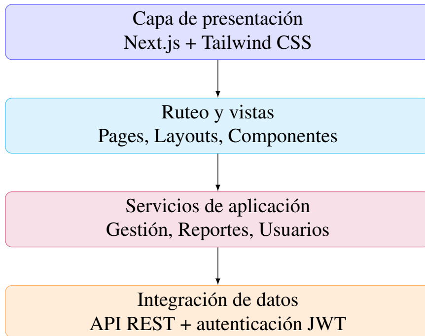
Figura 18. Arquitectura del panel web
