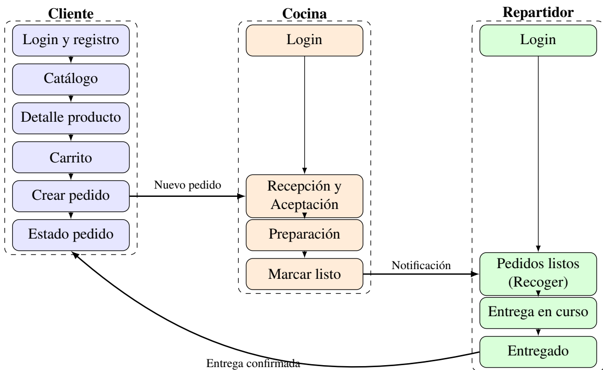
Figura 21. Flujo principal del frontend móvil para cliente, repartidor y cocina
