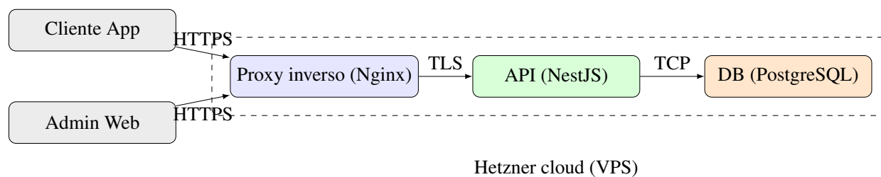
Figura 26. Arquitectura del despliegue de la plataforma
