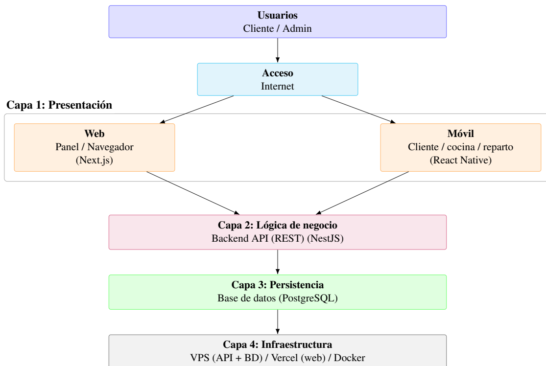
Figura 16. Arquitectura por capas de la plataforma SaaS
