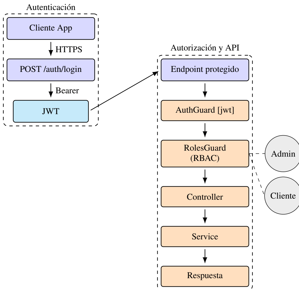
Figura 20. Flujo de autenticación y autorización (JWT + RBAC)
