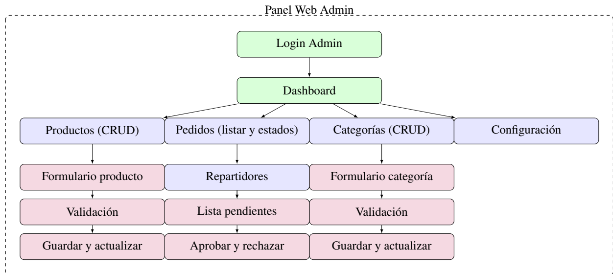
Figura 22. Flujo principal del panel web administrativo
