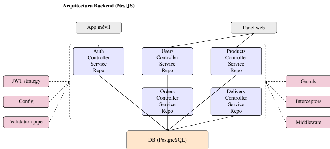
Figura 19. Arquitectura modular del backend (NestJS) planificada
