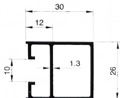
SECTION NO. - 70S-1501 EST. WEIGHT - 0.557 KG./M.
