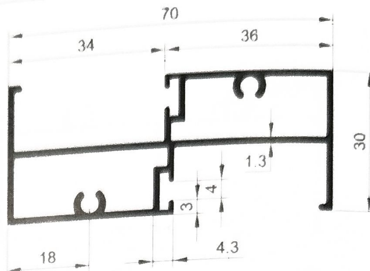
SECTION NO. - 70S - 1206 EST. WEIGHT - 0.916 KG./M.
