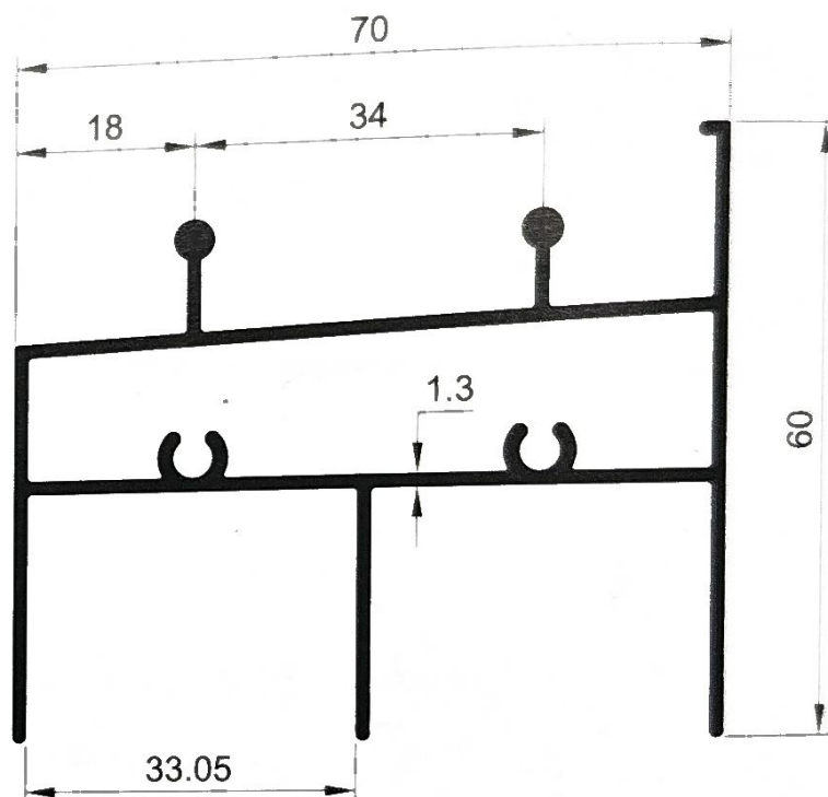
SECTION NO. - 70S - 1006 EST. WEIGHT - 1.118 KG./M.
