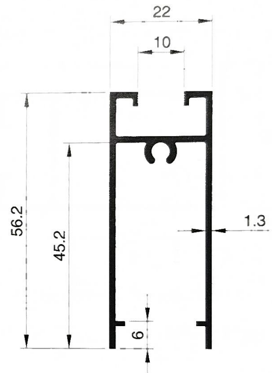
SECTION NO. - 70S-1501 EST. WEIGHT - 0.557 KG./M.
