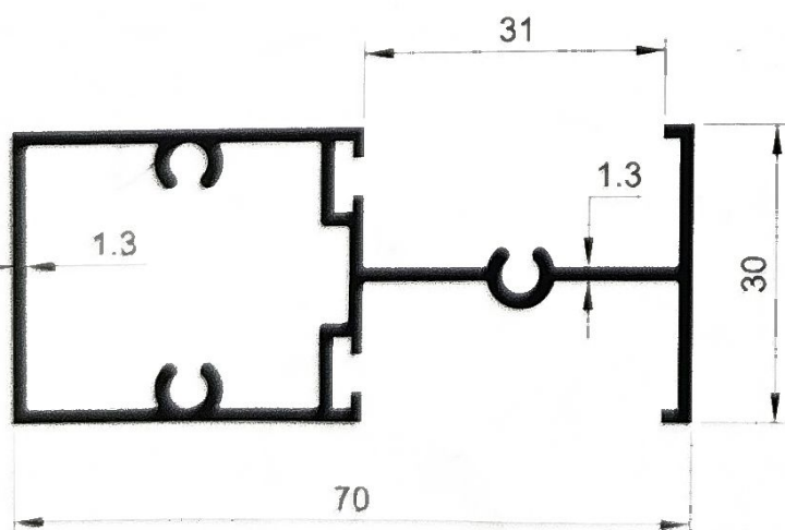
SECTION NO. - 70S - 1304 EST. WEIGHT - 0.831 KG./M.
