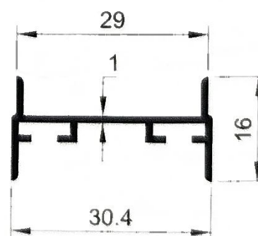
SECTION NO. - 70S - 1914 EST. WEIGHT - 0.199 KG./M.
