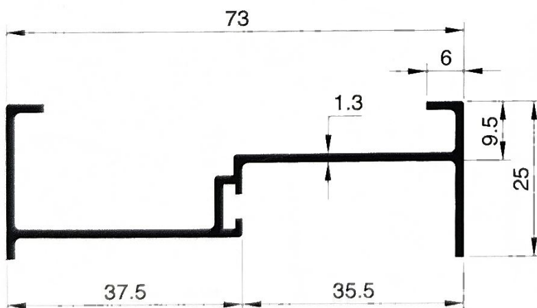
SECTION NO. - 70S - 1201 - 1 EST. WEIGHT - 0.518 KG./M.
