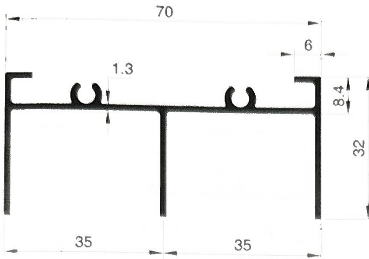
SECTION NO. - 70S - 1001-1 EST. WEIGHT - 0.664 KG./M.
