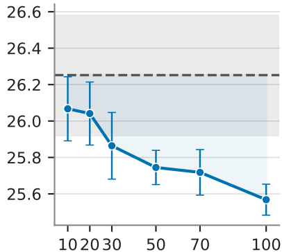
BrisT1D (n=15 patients)
