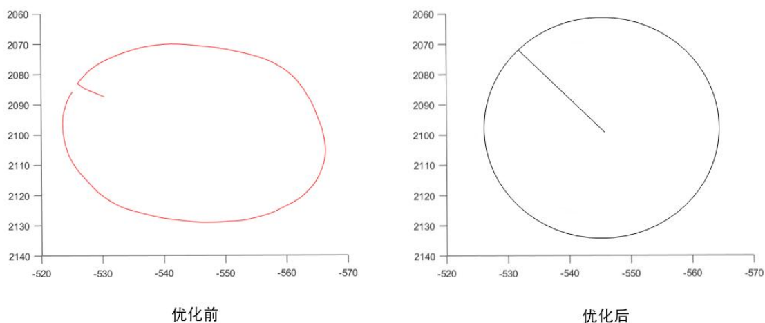
图 14 优化前后机器人圆轨迹跟踪对比
