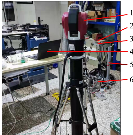
图 24 机构末端位置测量
