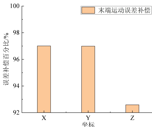
图 25 末端误差补偿百分比
