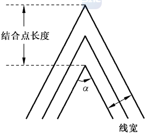
图 23 结合点长度
