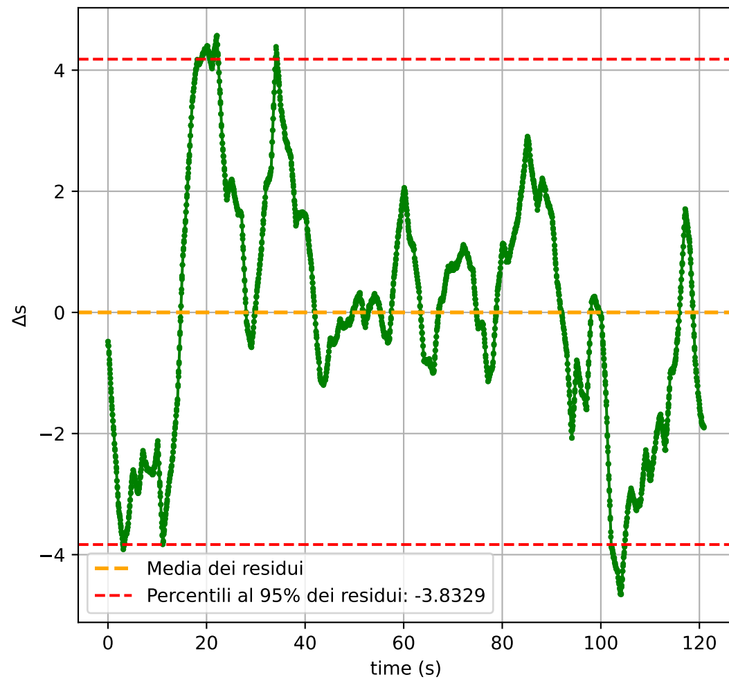
distribuzione dei residui
