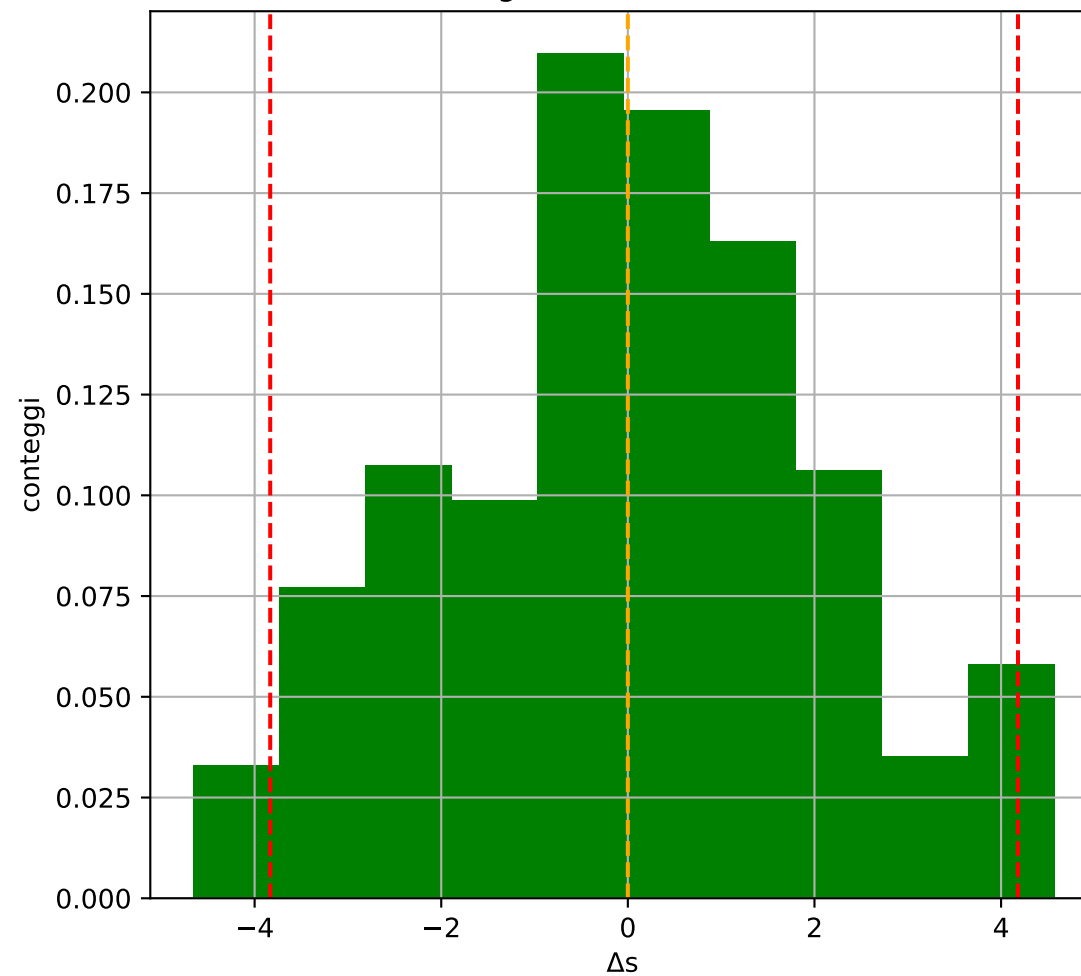
istogramma dei residui
