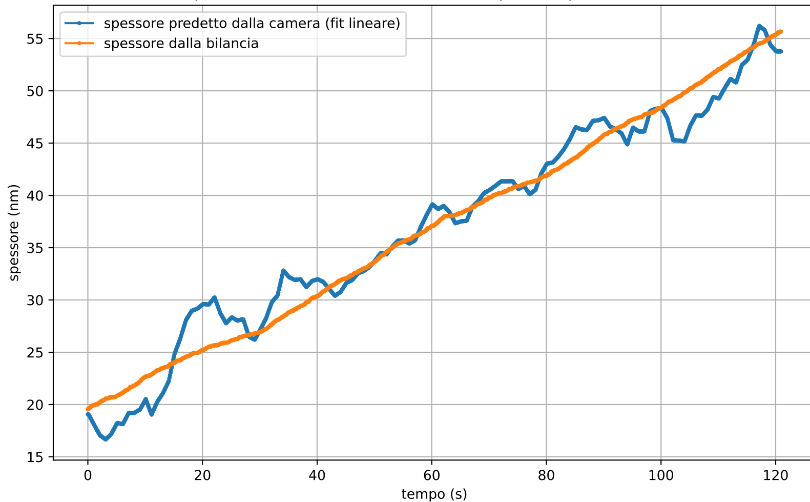
Confronto fra lo spessore misurato dalla bilancia e lo spessore predetto dai dati della camera
