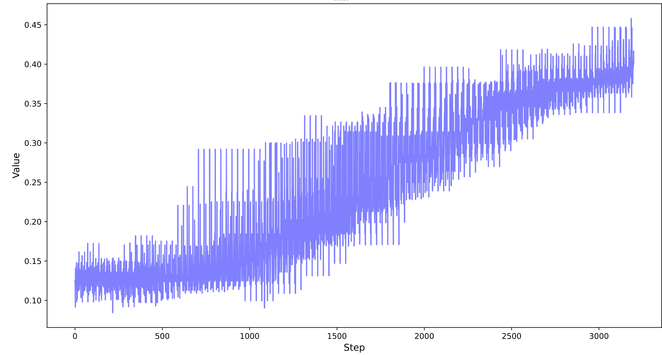
D_{mix} - NLO
