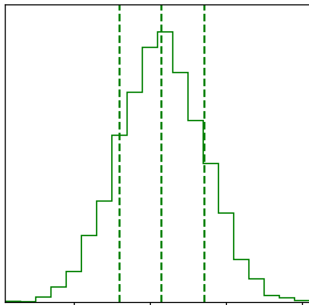
Corner Plot - LO
