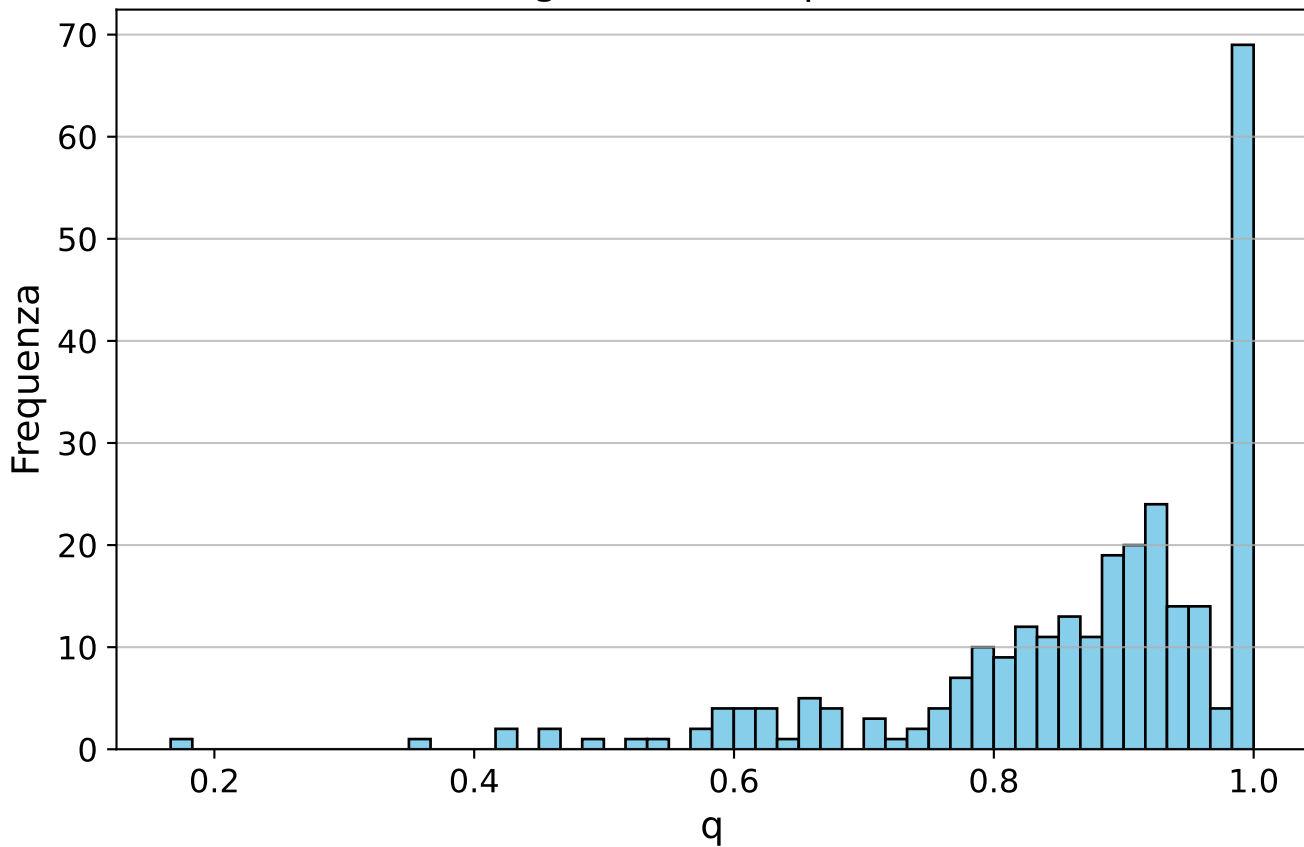
Istogramma dei q stimati
