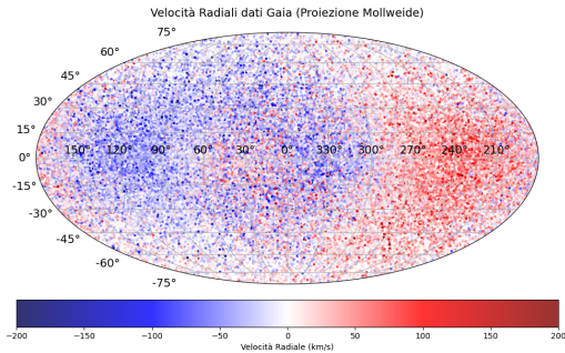
Figura 3: Mappa galattica (Proiezione Mollweide) delle velocità radiali ottenuta dai dati di Gaia .
