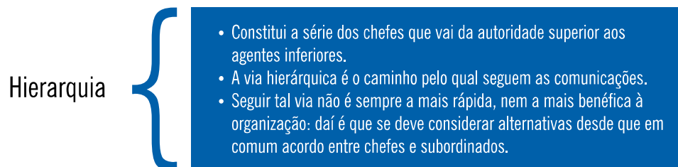
Figura 19: Hierarquia
