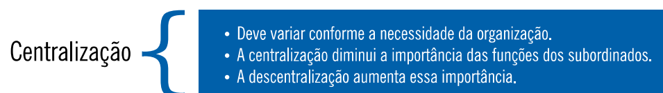
Figura 18: Centralização
