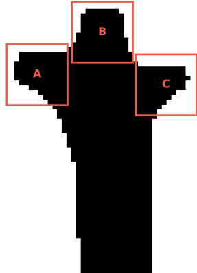
600-step gradient
