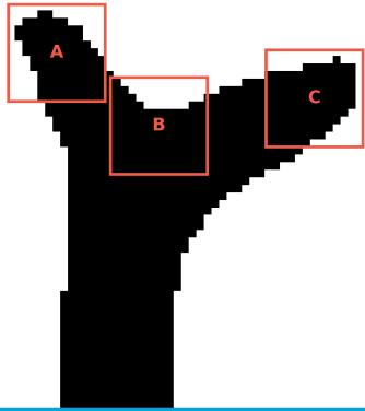
600-step gradient
