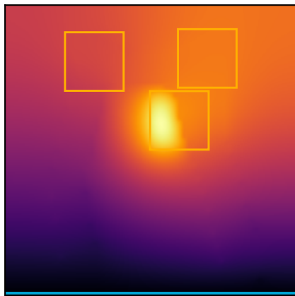
600-step gradient - scenario B Tmax=0.184093
