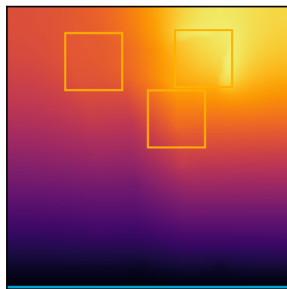
SENS U-Net + R25 - scenario C Tmax=0.175955
