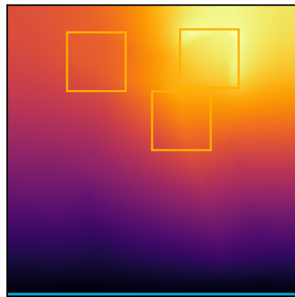
600-step gradient - scenario C Tmax=0.183564
