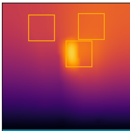
SENS U-Net + R25 - scenario B Tmax=0.164448
