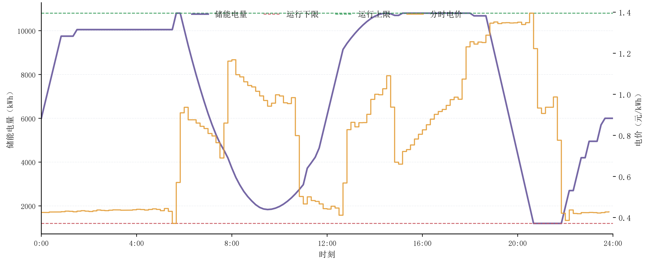
储能电量轨迹与分时电价
