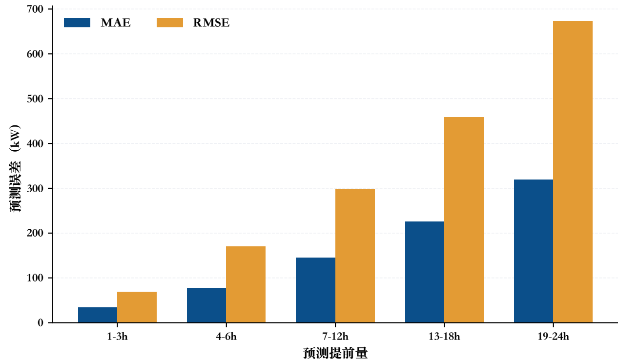
官方光伏预报误差随提前量的变化
