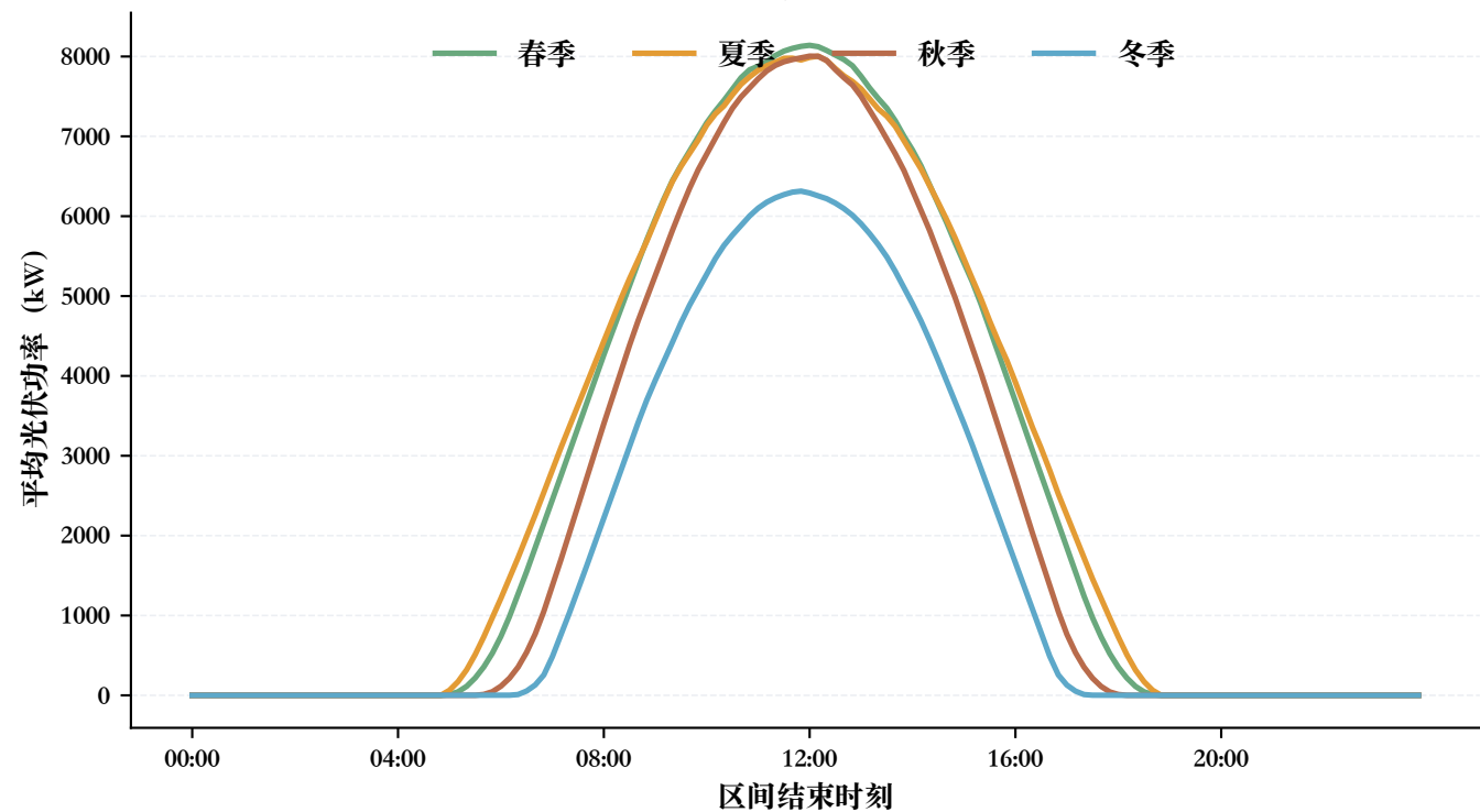
光伏出力的季节性日内轮廓
