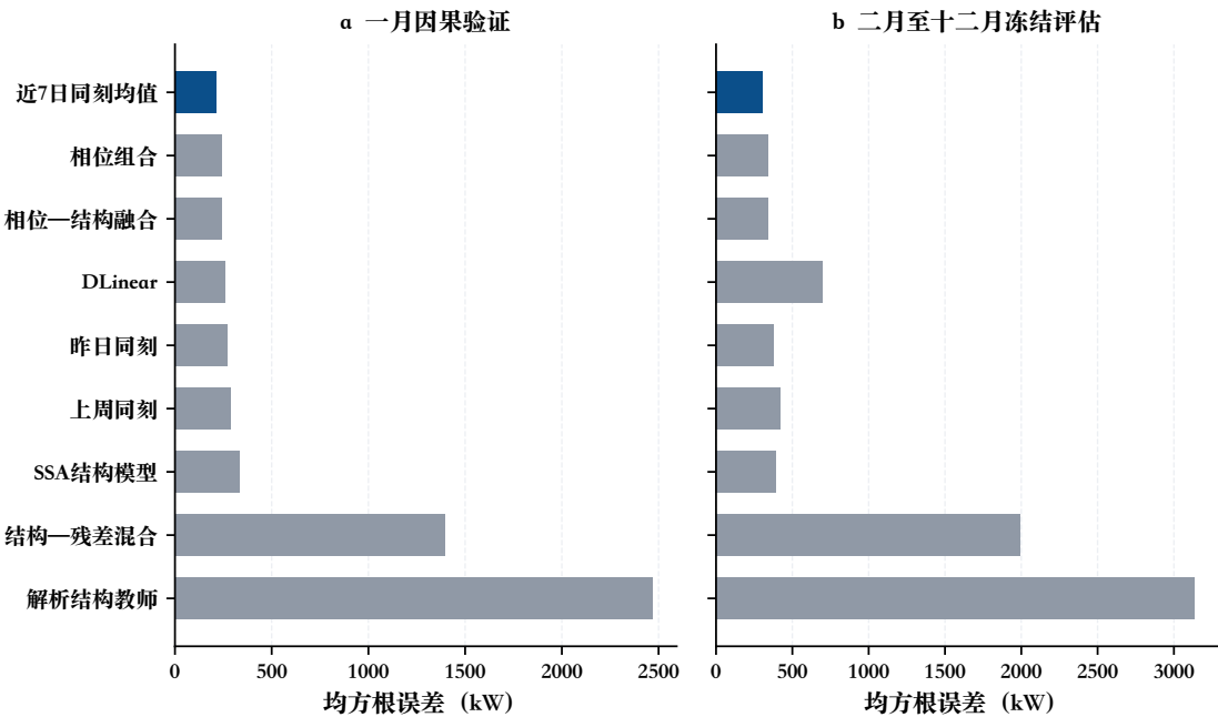
深蓝色仅表示由一月验证选定的正式模型；右图不参与模型选择。
