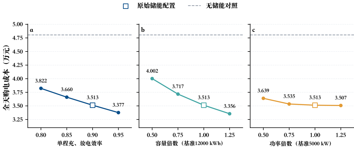
图 9 问题一储能物理参数的单因素灵敏度：连线仅连接已求解情形，方形标记为原始配置，虚线为无储能对照
