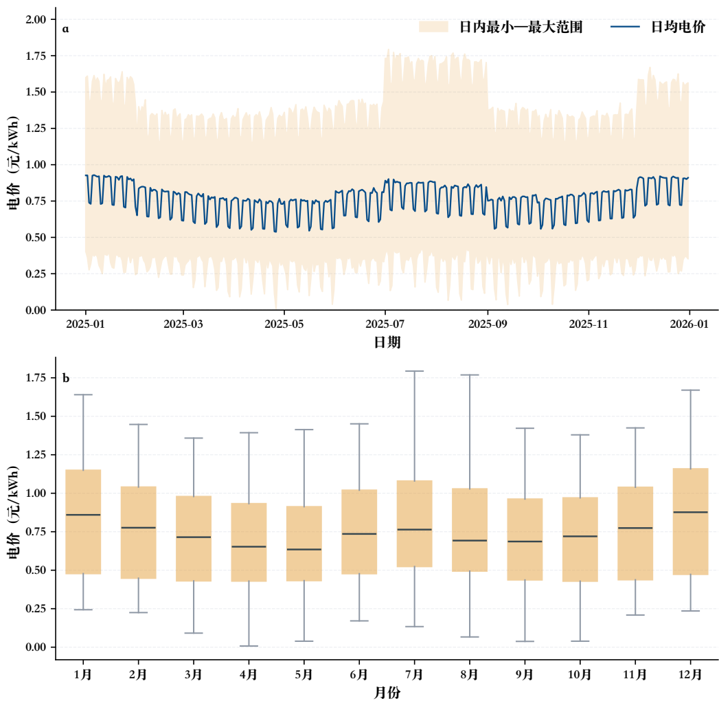
图 13 附件 4 动态电价的全年变化与月度分布
