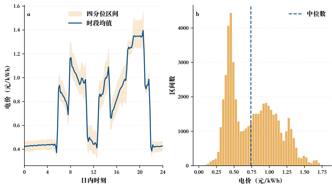
图 14 动态电价的日内轮廓与全年分布
