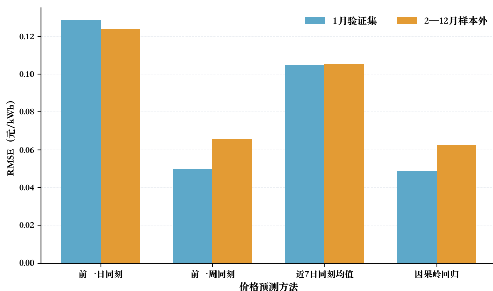
图 16 轻量因果电价预测方法的验证与样本外比较
