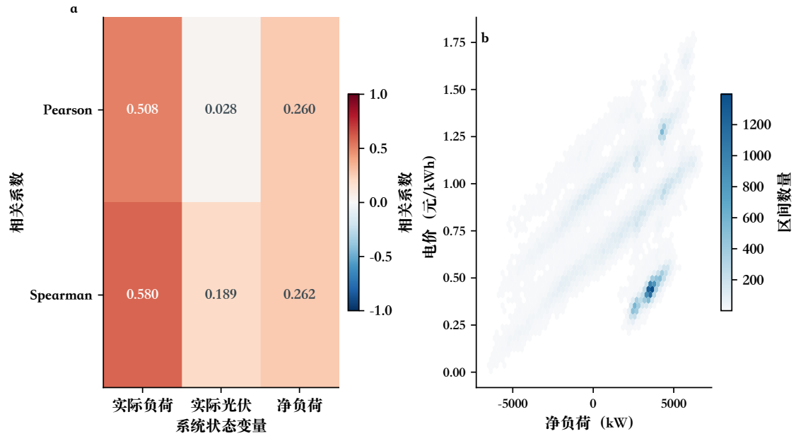
图 15 动态电价与负荷、光伏及净负荷的关联
